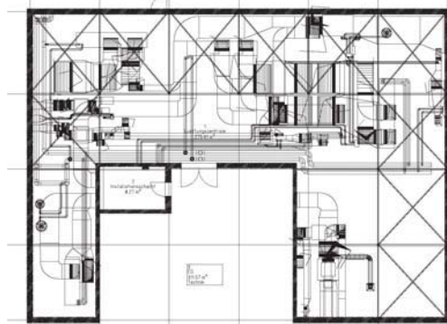
Grundriss
