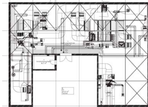
Grundriss
